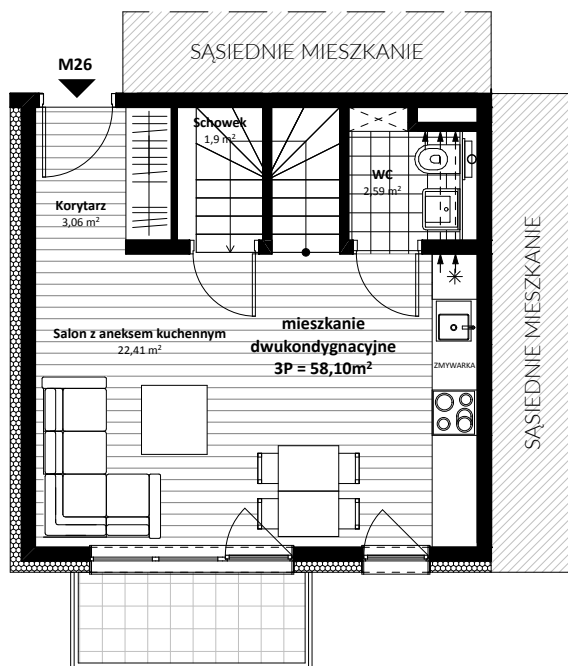
RZUT 1 PIĘTRA
